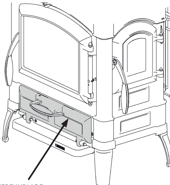
1 - ASCHESCHUBLADE
