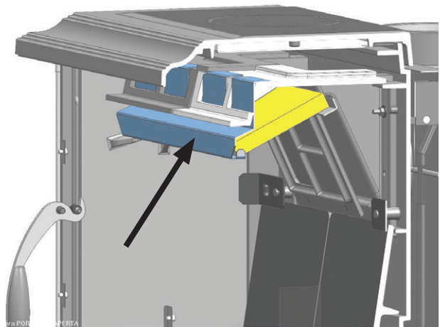
2 - RAUCHGASABWEISER
