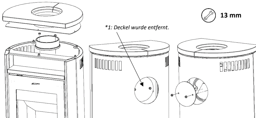
Abbildung 6 - Abgasstutzen und Abdeckung demontieren
