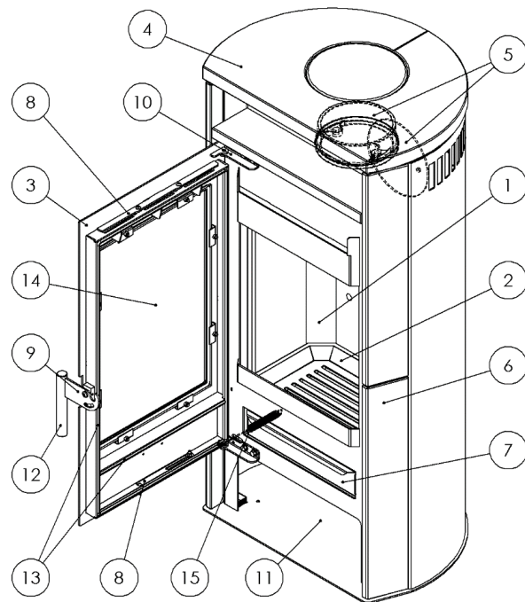
Abbildung 1 – Aufbau des Geräts
