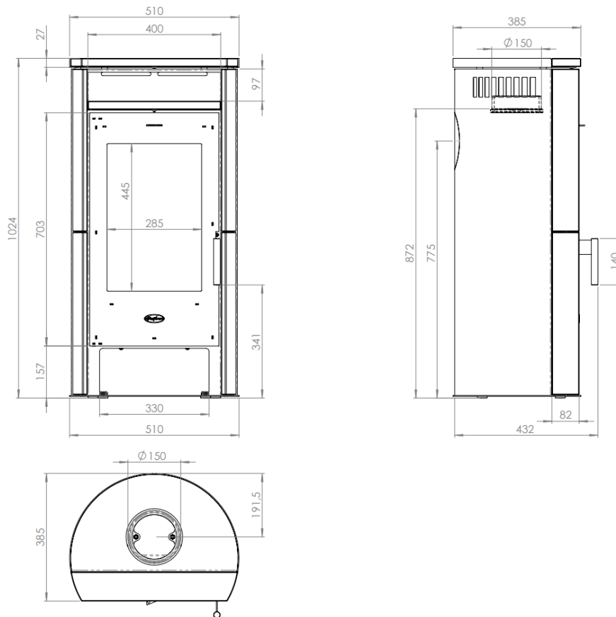
Abbildung 4 - Hauptmaße
