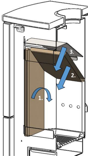
Abbildung 13 – Zugang zum Rauchraum
