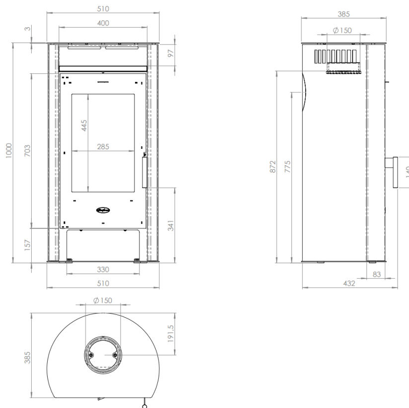
Abbildung 3 - Hauptmaße
