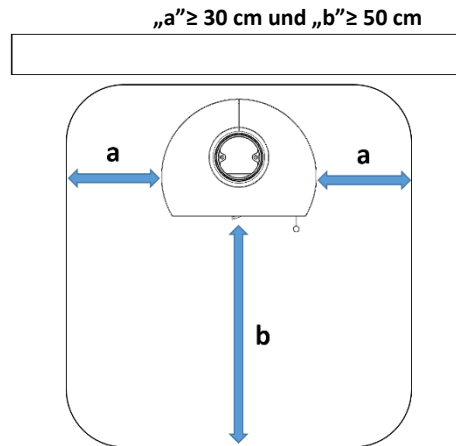
Abbildung 7 - Bodenplatte
