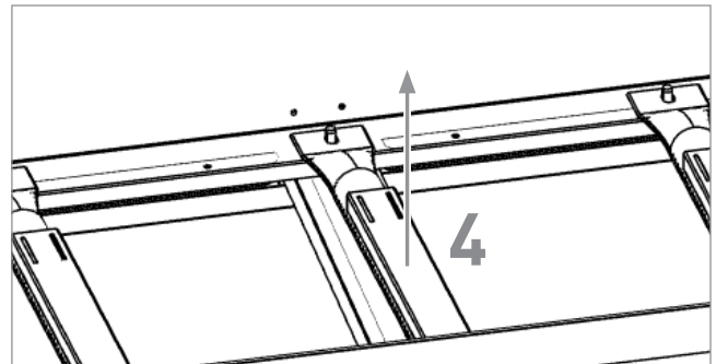
4 Nimm die Brenner aus der Brennkammer. Reinige den Brenner gründlich mit einer Nadel oder einem Pfeifenreiniger.
