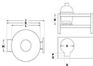
BOVENAANZICHT
