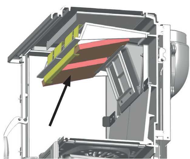
2 - RAUCHGASABWEISER
