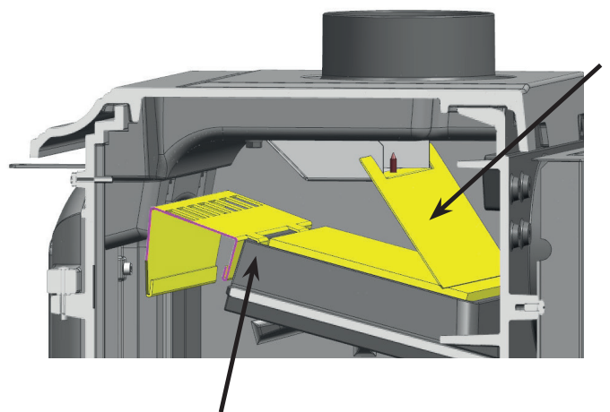
2 - RAUCHGASABWEISER
