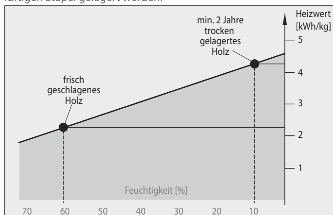
Abb. 2.1 Vergleich Heizwert trockenem Holz und frisch geschlagenem Holz Aus dem Diagramm geht hervor, dass der Verbrauch bei frisch geschlagenem Holz (Heizwert 2,3 kWh/kg) im Vergleich zu trockenem Holz (Heizwert 4,3 kWh/kg) fast doppelt so hoch ist.
