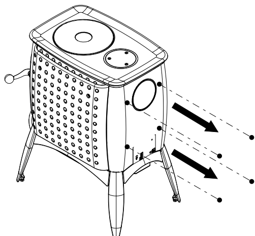
Abb. 18: Stiftschrauben heraus-schrauben
