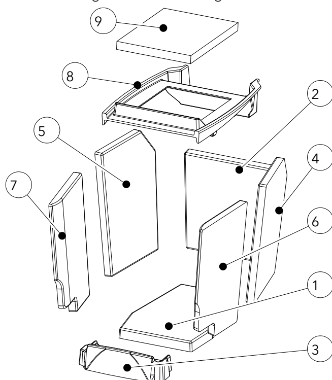
Abb. 23: Keramott einbauen
