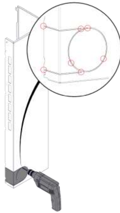
12) Löcher an den vorgesehenen Stellen bohren
