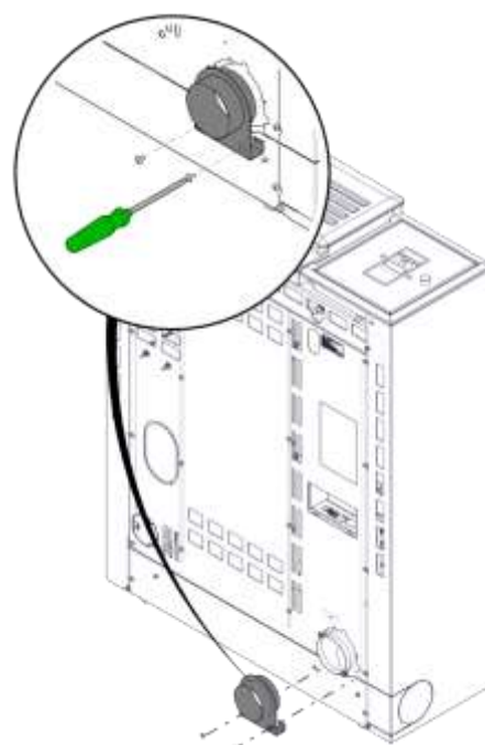
2) Den Halter abschrauben und entfernen
