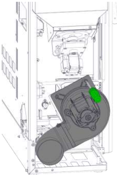
9) Den Ventilator komplett mit Rohr und Dichtung durch die anderen Löcher auf der Platte in die neue Position schrauben
