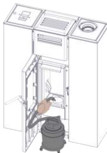
3) Asche absaugen
