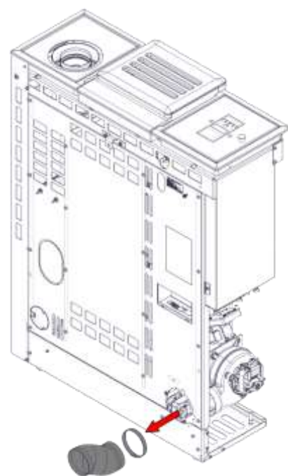
6) Schelle und Rohr entfernen
