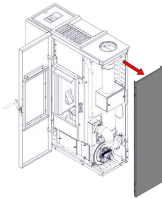
6) Seitenwand entfernen
