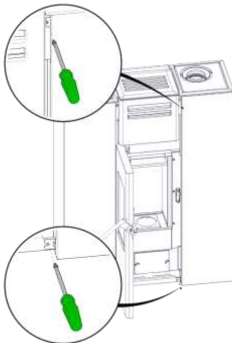
2) Schrauben abschrauben
