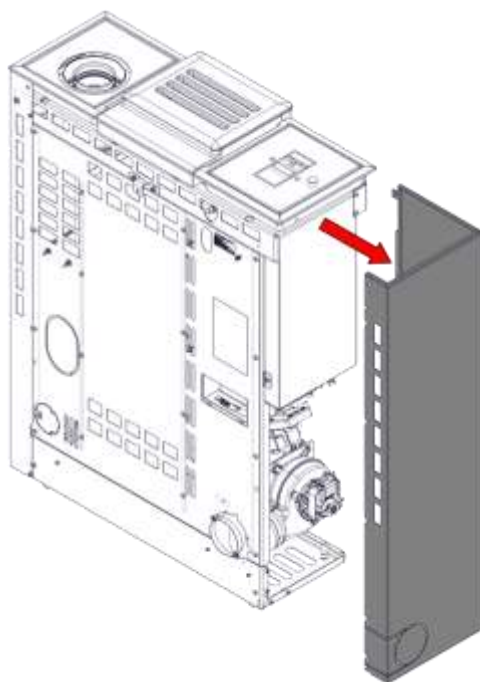
5) Seitenwand entfernen
