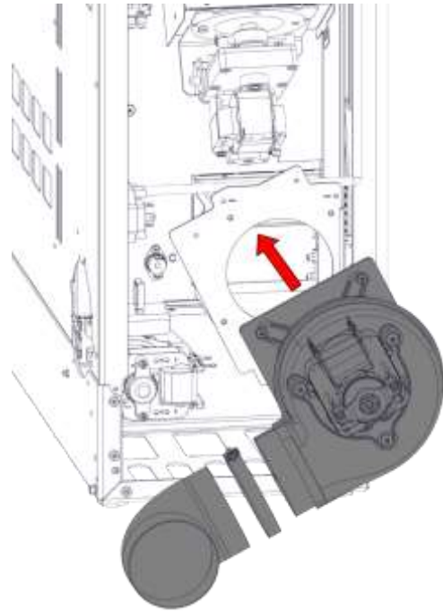
8) Die zuvor entfernte Schelle und das Rohr einsetzen
