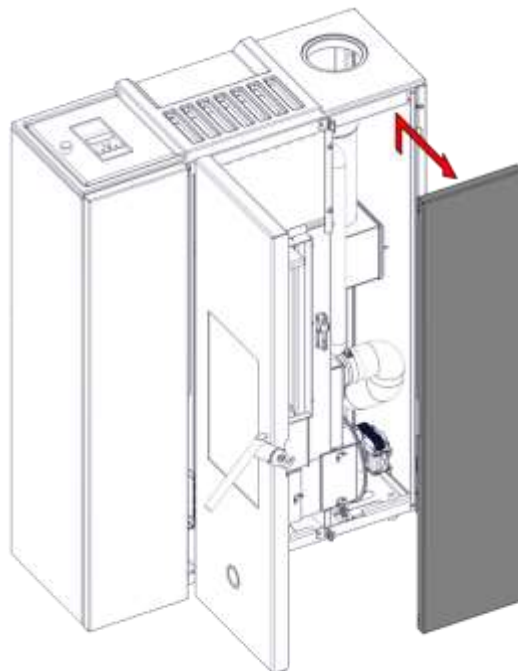
3) Die Frontplatte entfernen
