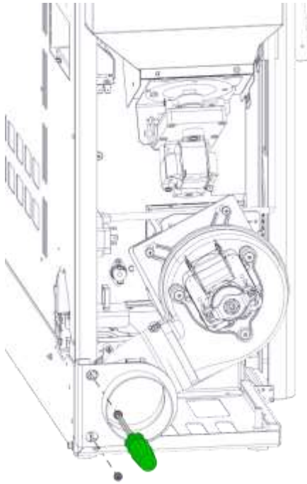
11) Halterung anschrauben
