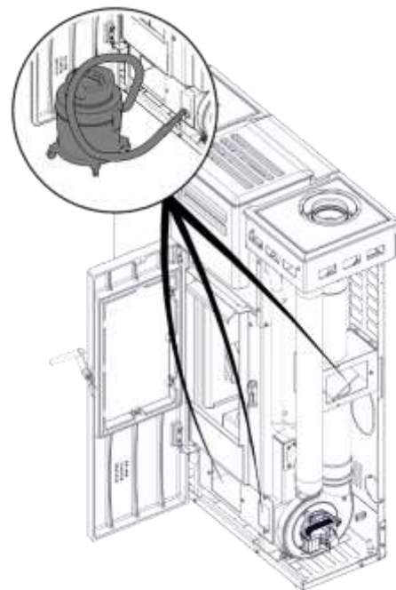
6) Die Kammern absaugen
