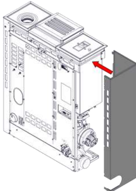
14) Die zuvor demontierte Seitenwand wieder zusammenbauen
