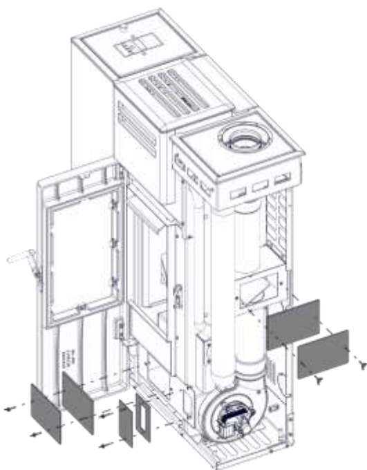
7) Inspektionen abschrauben und entfernen
