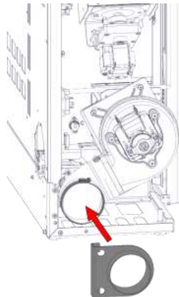
8) Die zuvor entfernte Schelle und das Rohr einsetzen
