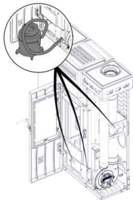
8) Die Kammern absaugen
