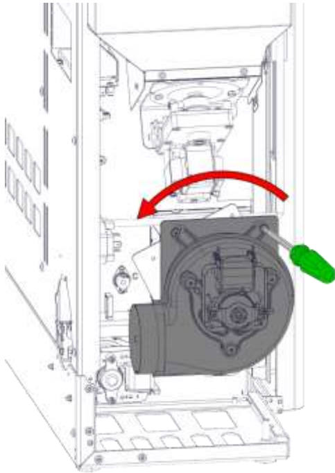
7) Ventilator und Dichtung von der Platte abschrauben und drehen
