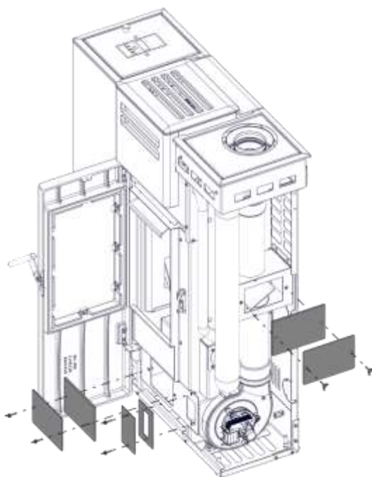
5) Inspektionen abschrauben und entfernen
