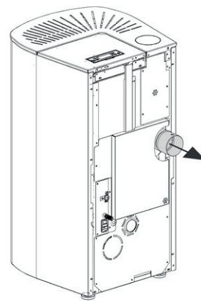
OPTIONALES ZUBEHÖR (90°-Bogen) HINTERER RAUCHAUSLASS
