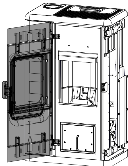
Abb. 100: Tür öffnen
