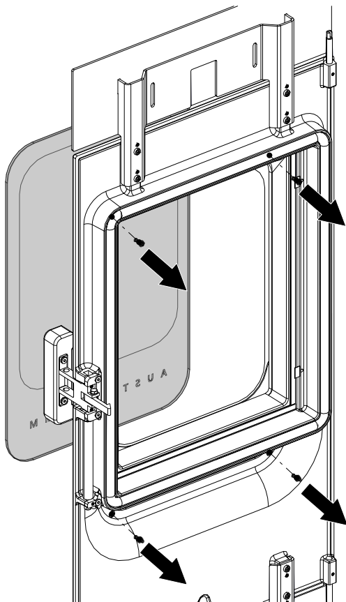
Abb. 103: Dekoglas abnehmen
