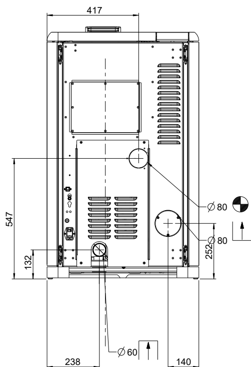
Abb. 46: Abmessungen
