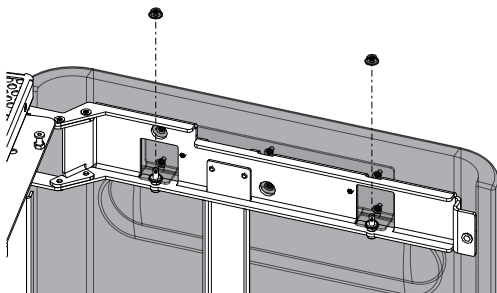
Abb. 36: Keramikverkleidung anbringen
