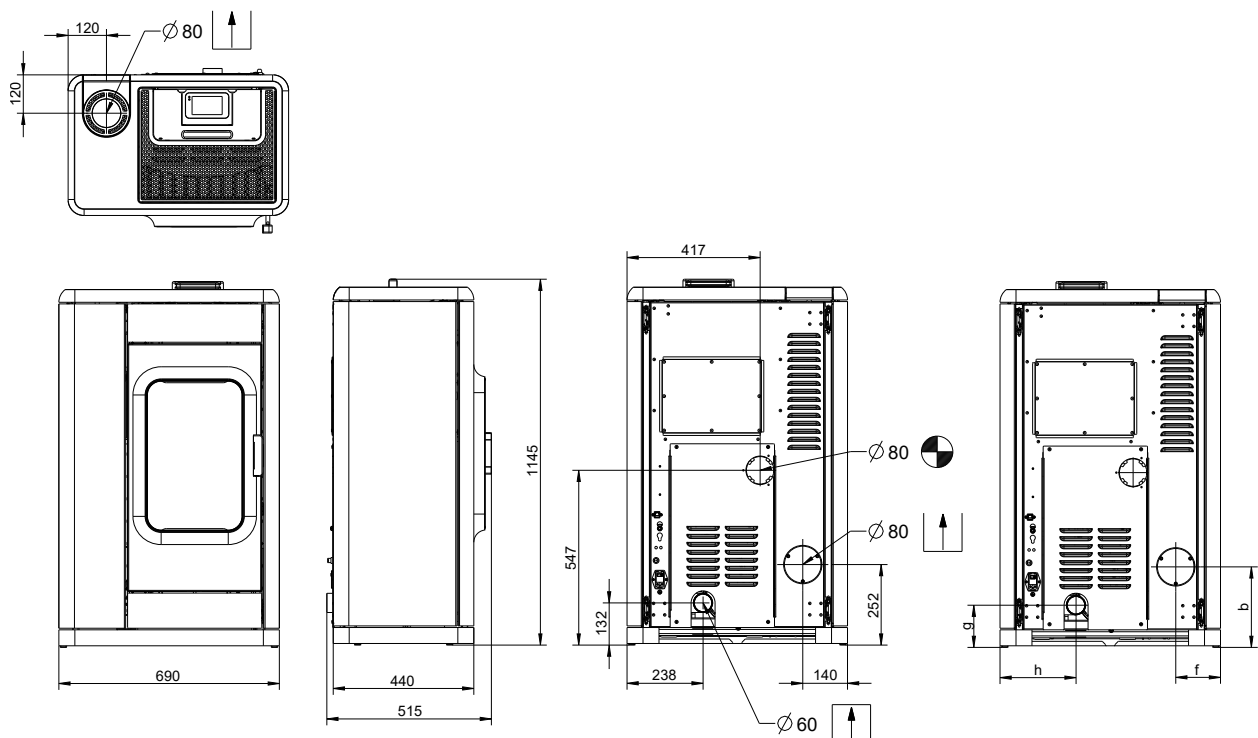
Abb. 2: Ruby Abmessungen
