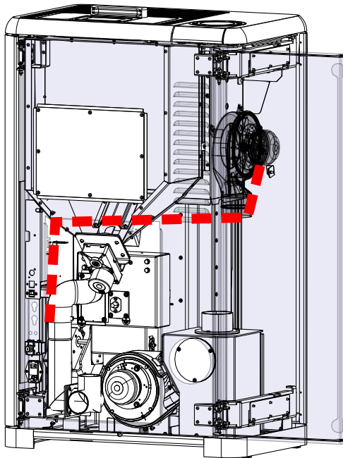
Abb. 22: Kabel durchziehen
