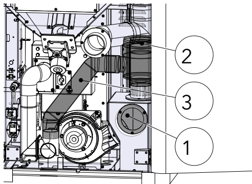
Abb. 14: Poujoulat montieren
