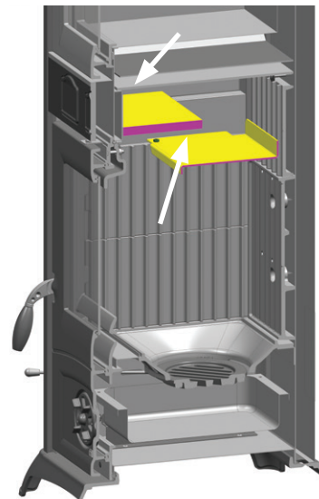
2 - RAUCHGASABWEISER
