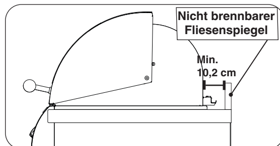
Abb. 10-4 Freiraum bei Fliesenspiegel
