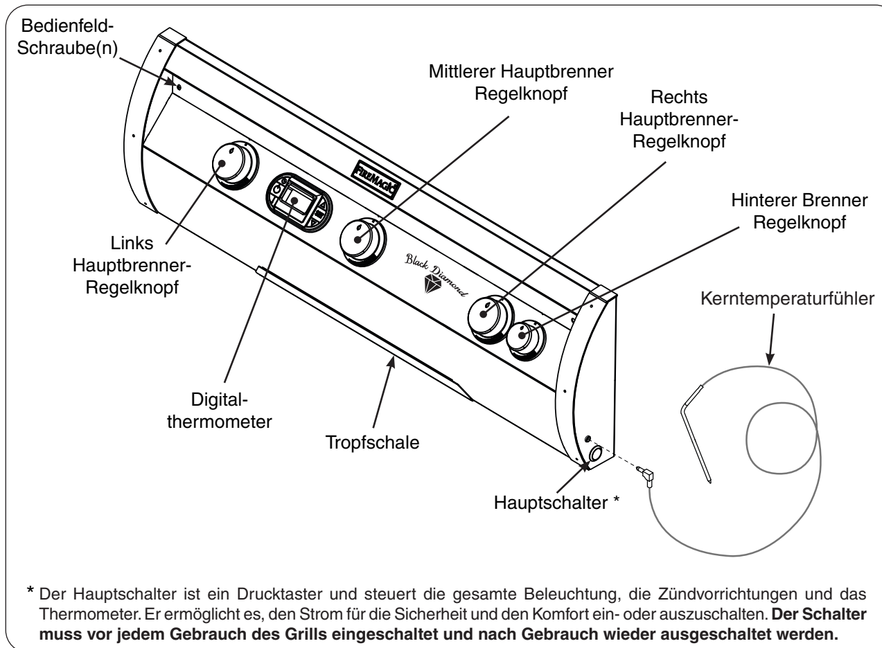
Abb. 26-1 H790i Bedienelemente
