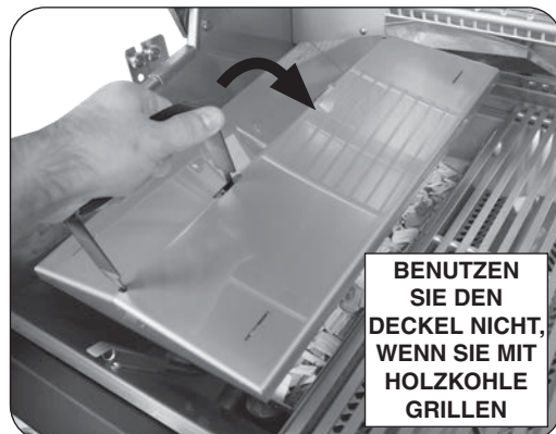
Abb. 34-5 Räucherofendeckel montieren
