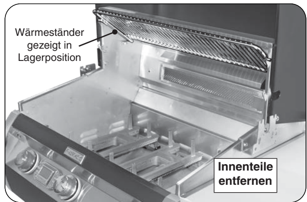
Abb. 32-1 Bereiten Sie den Grill zum Rotieren vor
