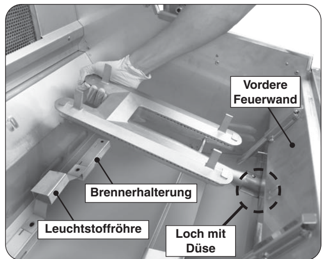
Abb. 40-2 Brenner ausbauen
