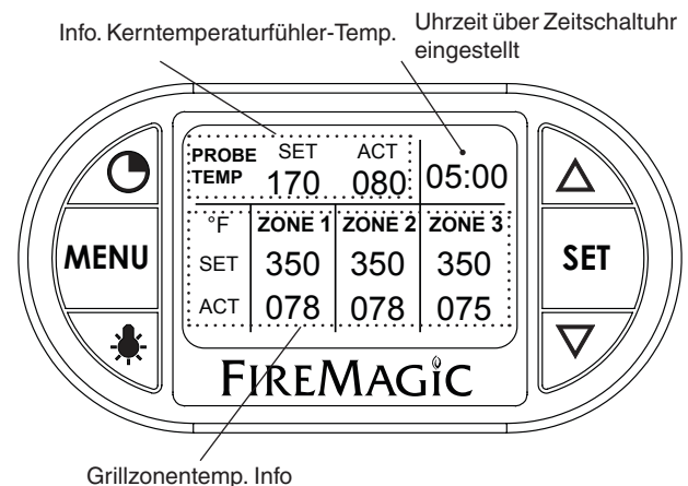
Abb. 29-3 Standard-Bildschirmdetail
