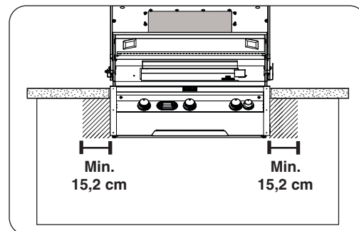
Abb. 11-1 Bedienfeldabstände
