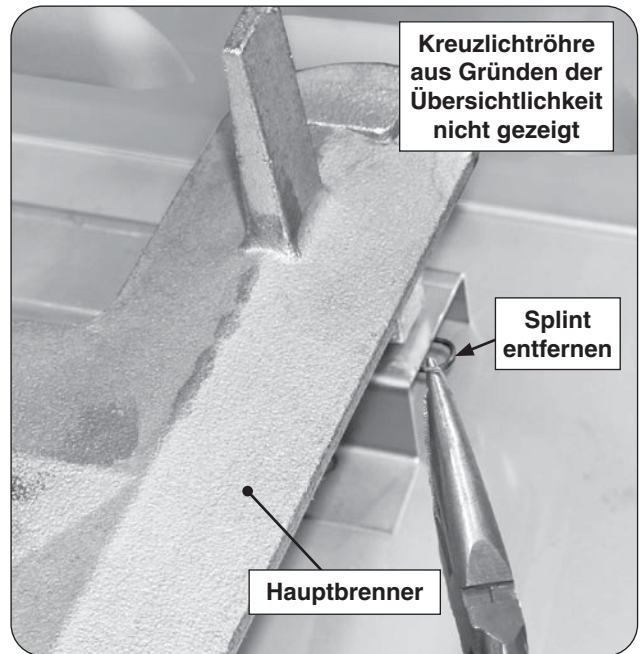
Abb. 40-1 Hauptbrenner ausbauen
