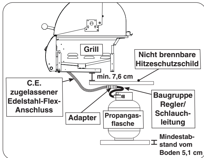
Abb. 8-1 Anordnung Propangasflasche
