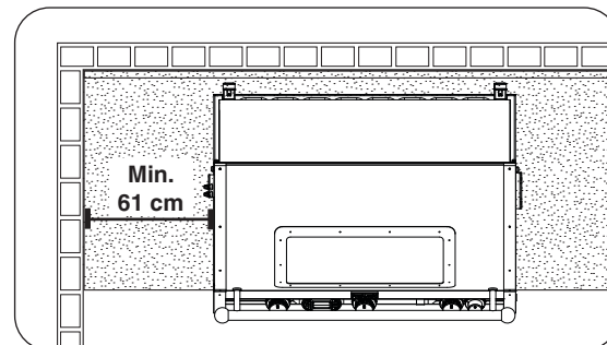
Abb. 10-5 Seiten- / Eckwandabstand
