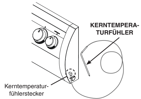
Abb. 29-1 Kerntemperaturfühlerdetails
