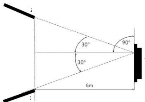
Abb. 51: Betriebswinkel
