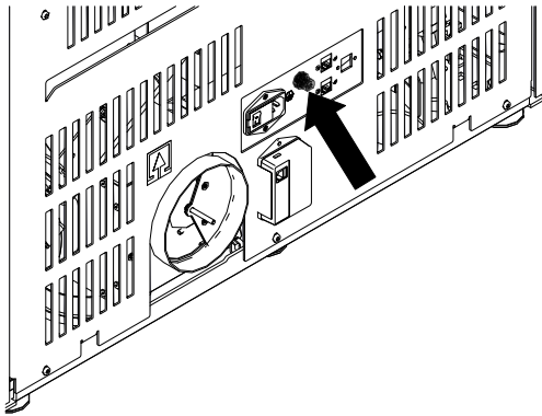
Abb. 104: Sicherheitstemperaturbegrenzer
