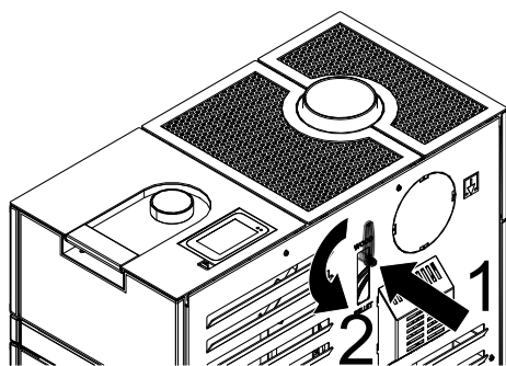
Abb. 43: Rauchgasklappe schließen
