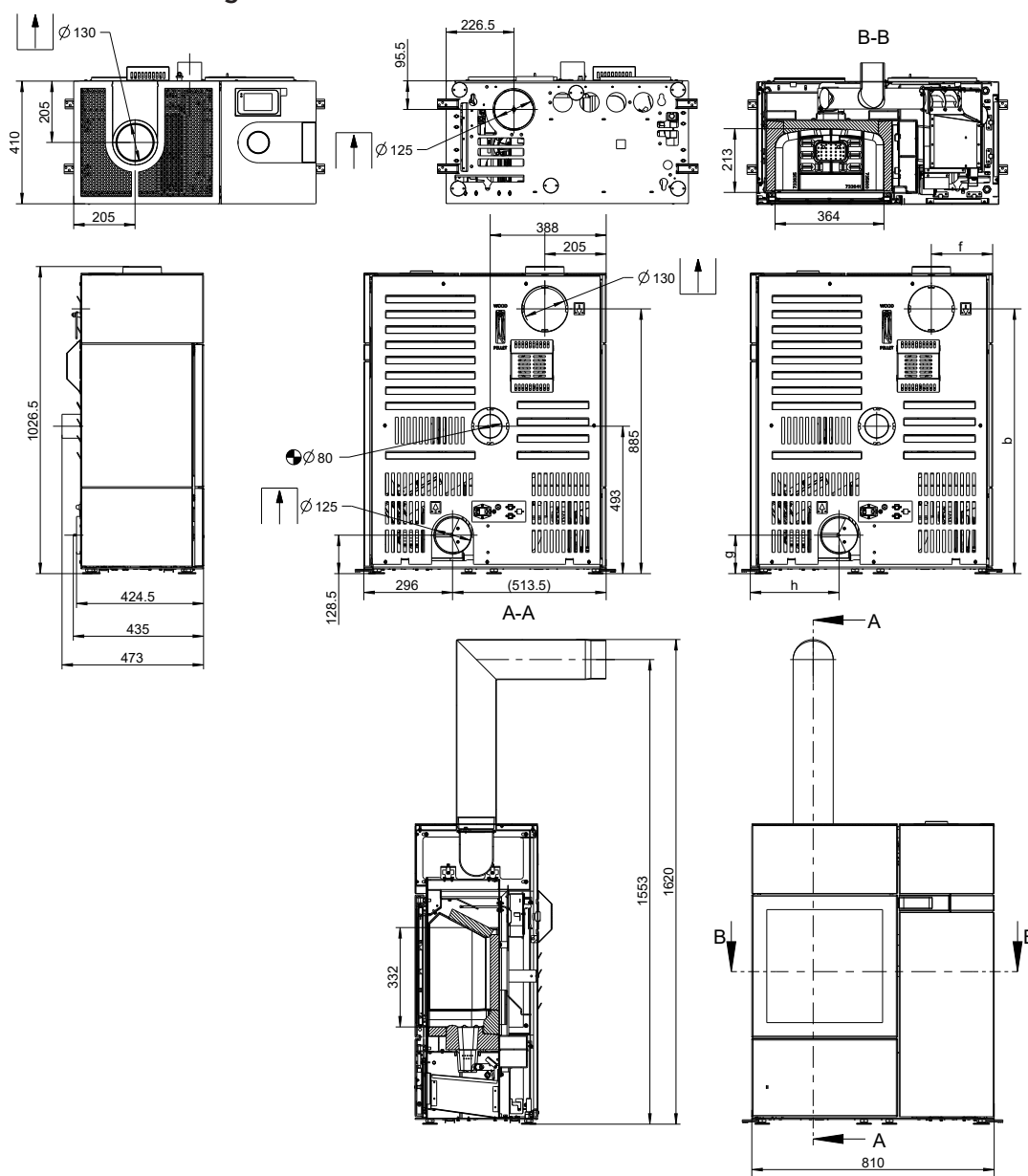
Abb. 2: Abmessungen
