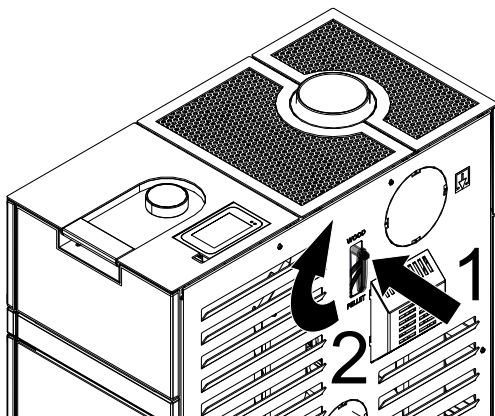
Abb. 47: Rauchgasklappe öffnen
