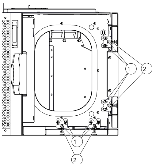
Abb. 15: Verkleidung einstellen
