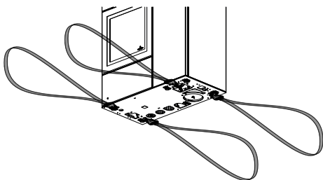
Abb. 7: Transporthilfe
