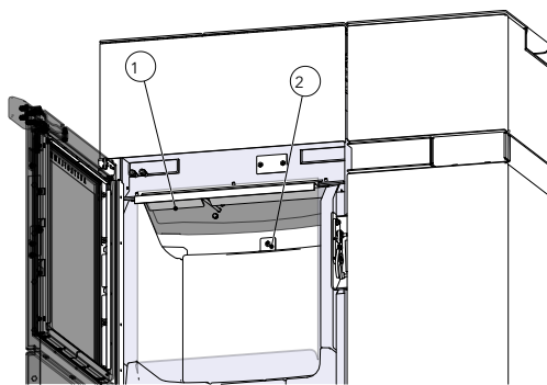
Abb. 93: Zugplatte anheben
