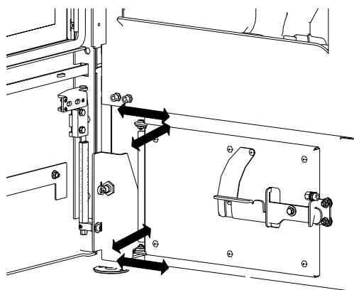
Abb. 80: Ascheladentür einstellen
