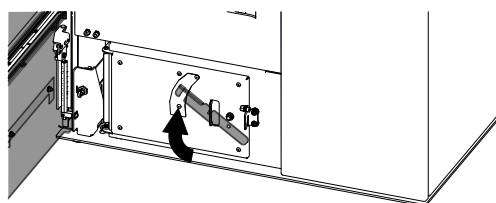
Abb. 86: Aschenladetür öffnen
