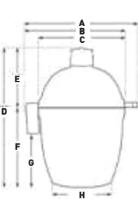
VISTA LATERAL
