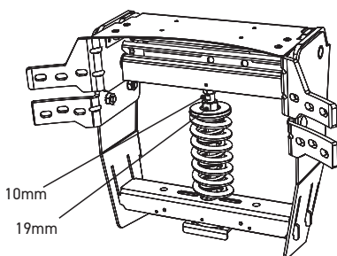
BISAGRA ALTERNATIVA
