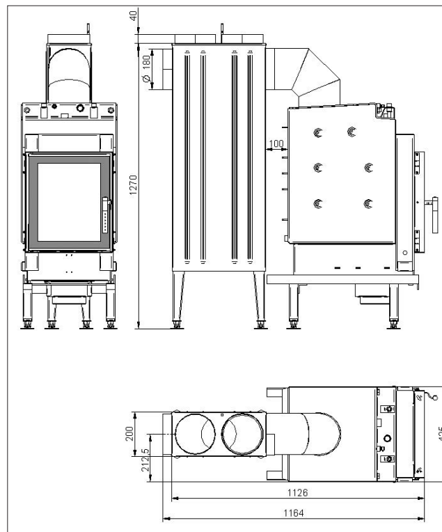
Abb. 1d Renova A H 2 O mit Nachschaltheizfläche
