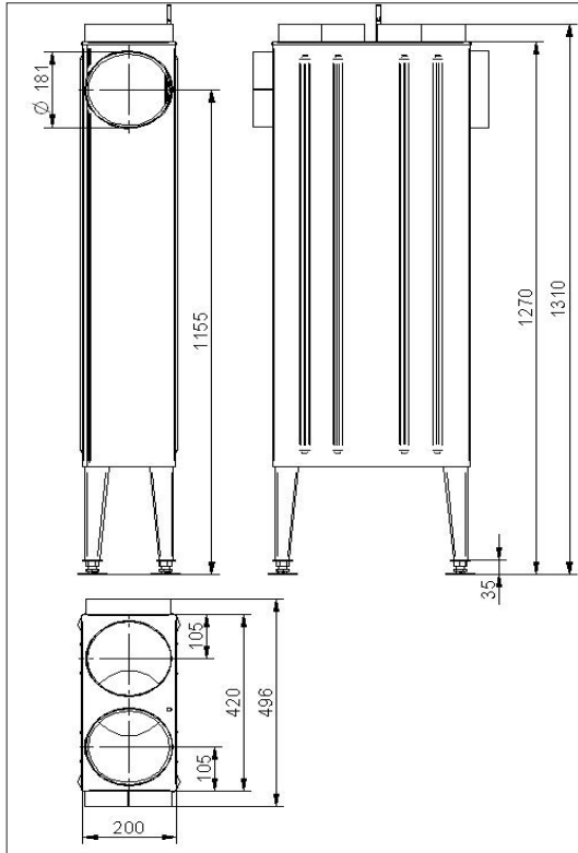
Abb. 1e Nachschalttheizfläche
