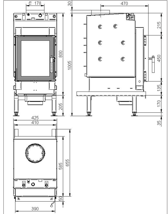
Abb. 1b Renova A H 2 O mit Zarge für Frontblende
