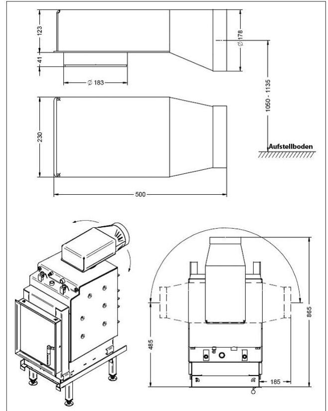
Abb. 1f Abgasanschluss flach
