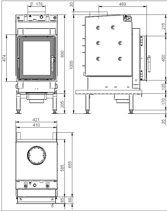
Abb. 1a Renova A H 2 O mit Mauerhals
