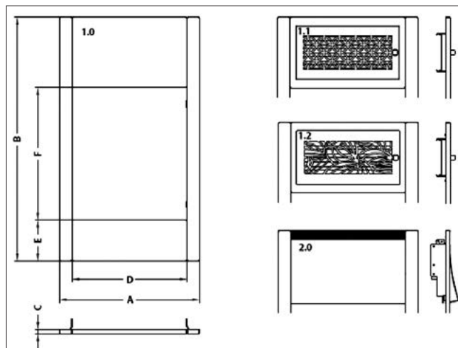
Abb. 1c Frontblenden
