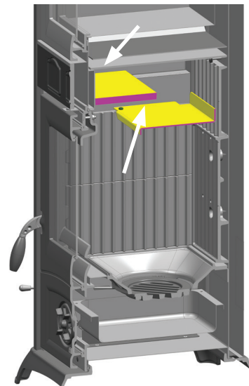
2 - RAUCHGASABWEISER
